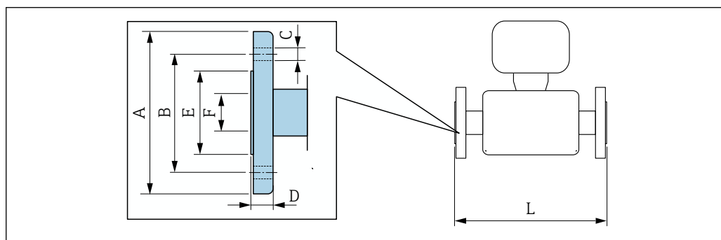
Подвижный фланец, штампованная пластина
