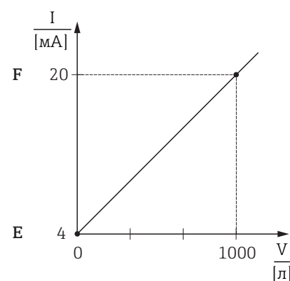
Рис. 32: Калибровка по эталонному давлению – калибровка «мокрого» типа
