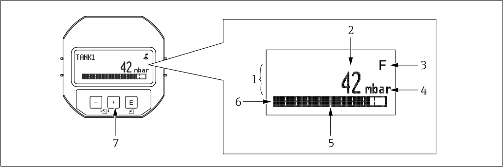
Рис. 28: Индикация 1 Основная строка 2 Значение 3 Символ 4 Единица измерения 5 Гистограмма 6 Информационная строка 7 Кнопки управления
