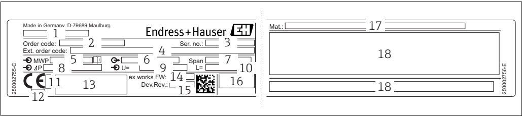
Рис. 1: Заводская табличка
