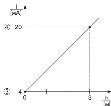
Рис. 4: Калибровка по эталонному давлению – калибровка «мокрого» типа
