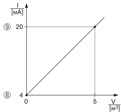
Рис. 18: Калибровка 2-й измеряемой переменной
