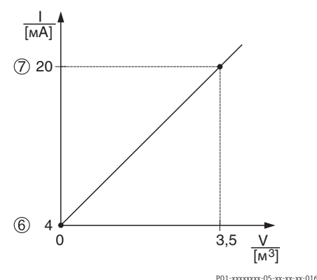
Рис. 15: Полуавтоматический ввод таблицы линейаризации
