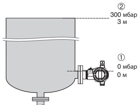
Рис. 3: Калибровка по эталонному давлению – калибровка «мокрого» типа
