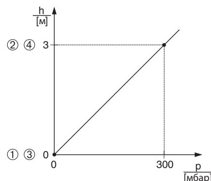
Рис. 17: Калибровка 1-й измеряемой переменной
