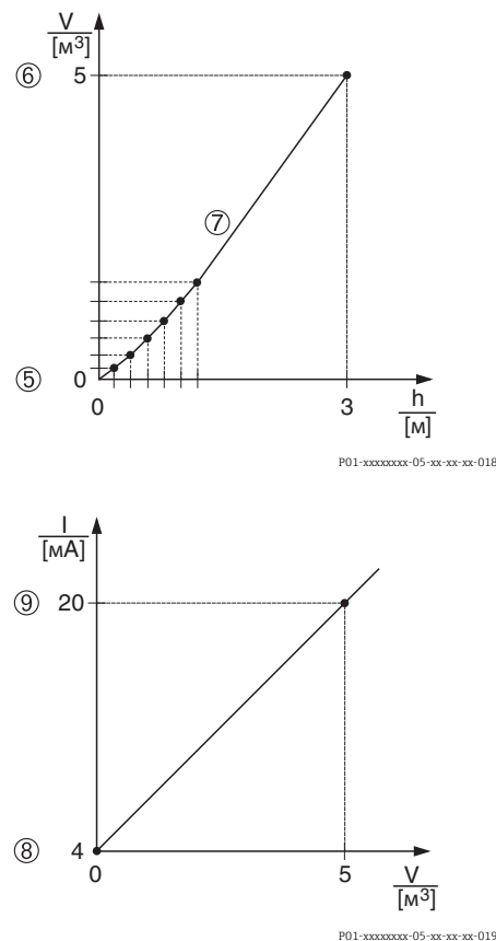
Рис. 19: Калибровка 2-й измеряемой переменной
