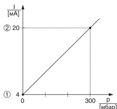
Рис. 1: Калибровка по эталонному давлению
