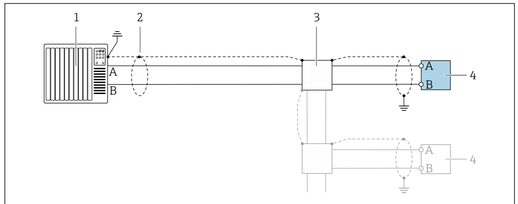
8 Пример подключения для Modbus RS485, безопасная зона и зона 2/разд. 2
