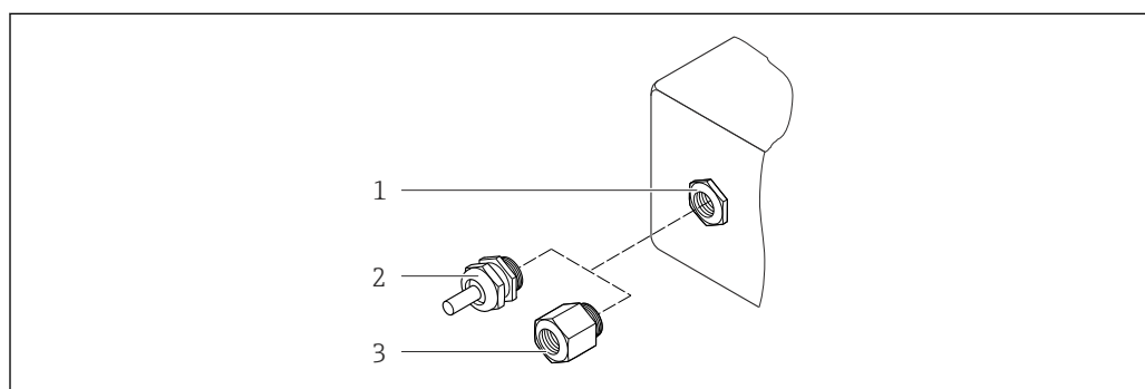
28 Доступные кабельные вводы/кабельные уплотнители
