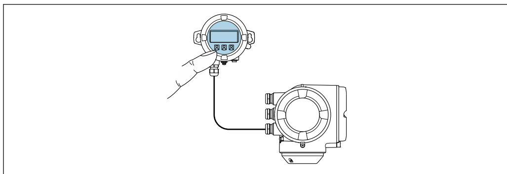
30 Управление с помощью выносного дисплея и модуля управления DKX001
