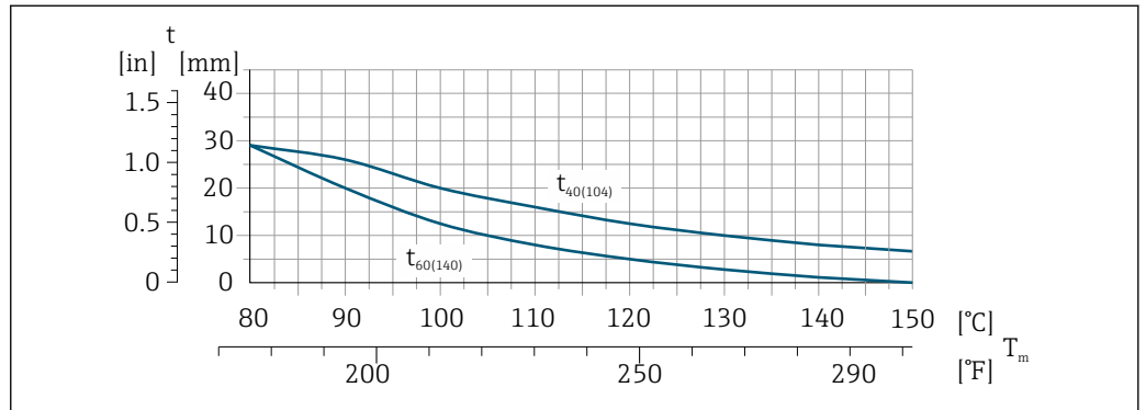
6 Рекомендованная максимальная толщина изоляции ( t ) зависит от температуры среды ( T ) и температуры окружающей среды ( T_a )
