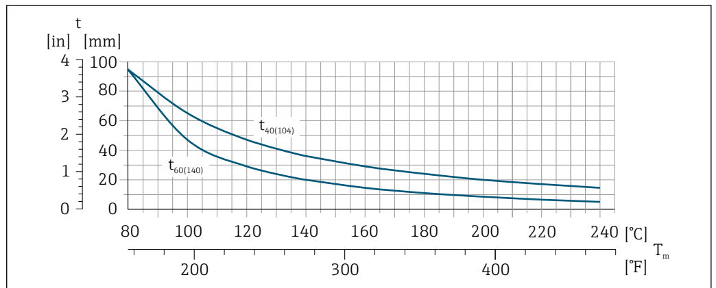
7 Рекомендованная максимальная толщина изоляции ( t ) зависит от температуры среды ( T ) и температуры окружающей среды ( T_a )
