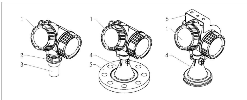
1 Конструкция уровнемера Micropilot FMR50 (26 ГГц)
