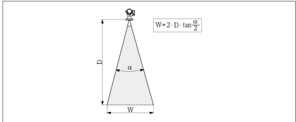
4 Зависимость между углом луча \alpha , расстоянием D и диаметром луча W
