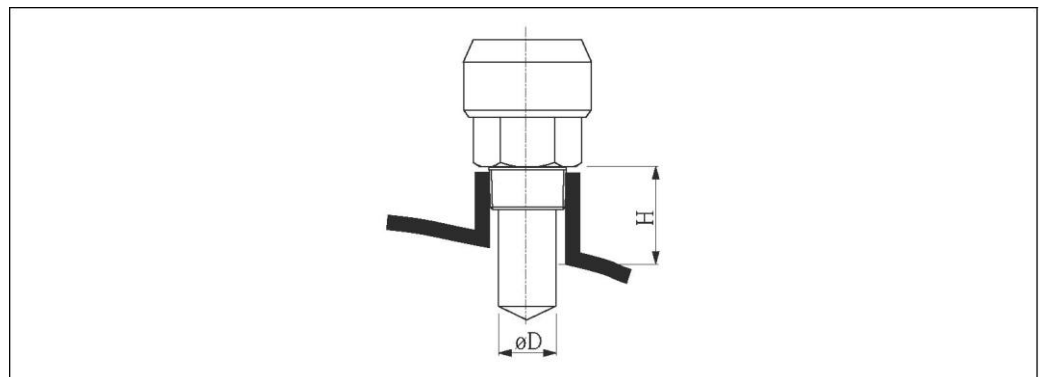
5 Высота патрубка и диаметр рупорной антенны с оболочкой (FMR50)
