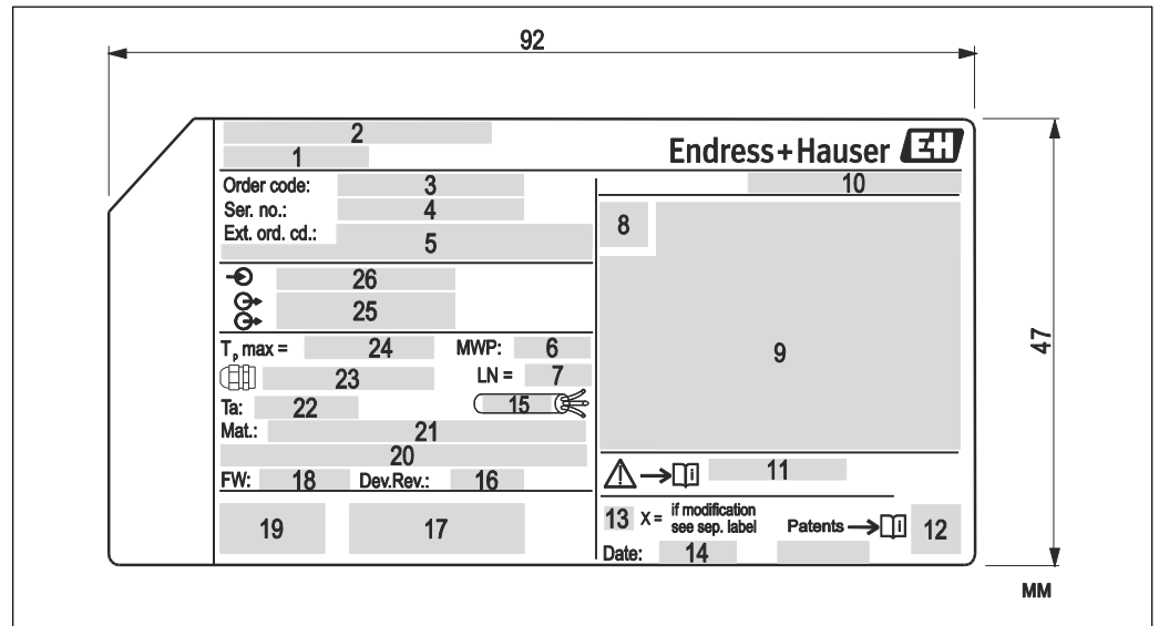
3 Заводской шильдик уровнемера Micropilot
